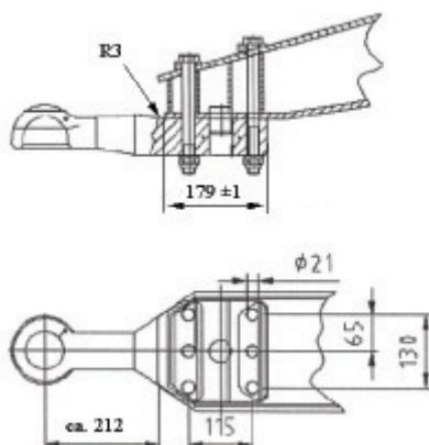
Abb. 1: Anbaubeispiele mit Anschlussmaßen
