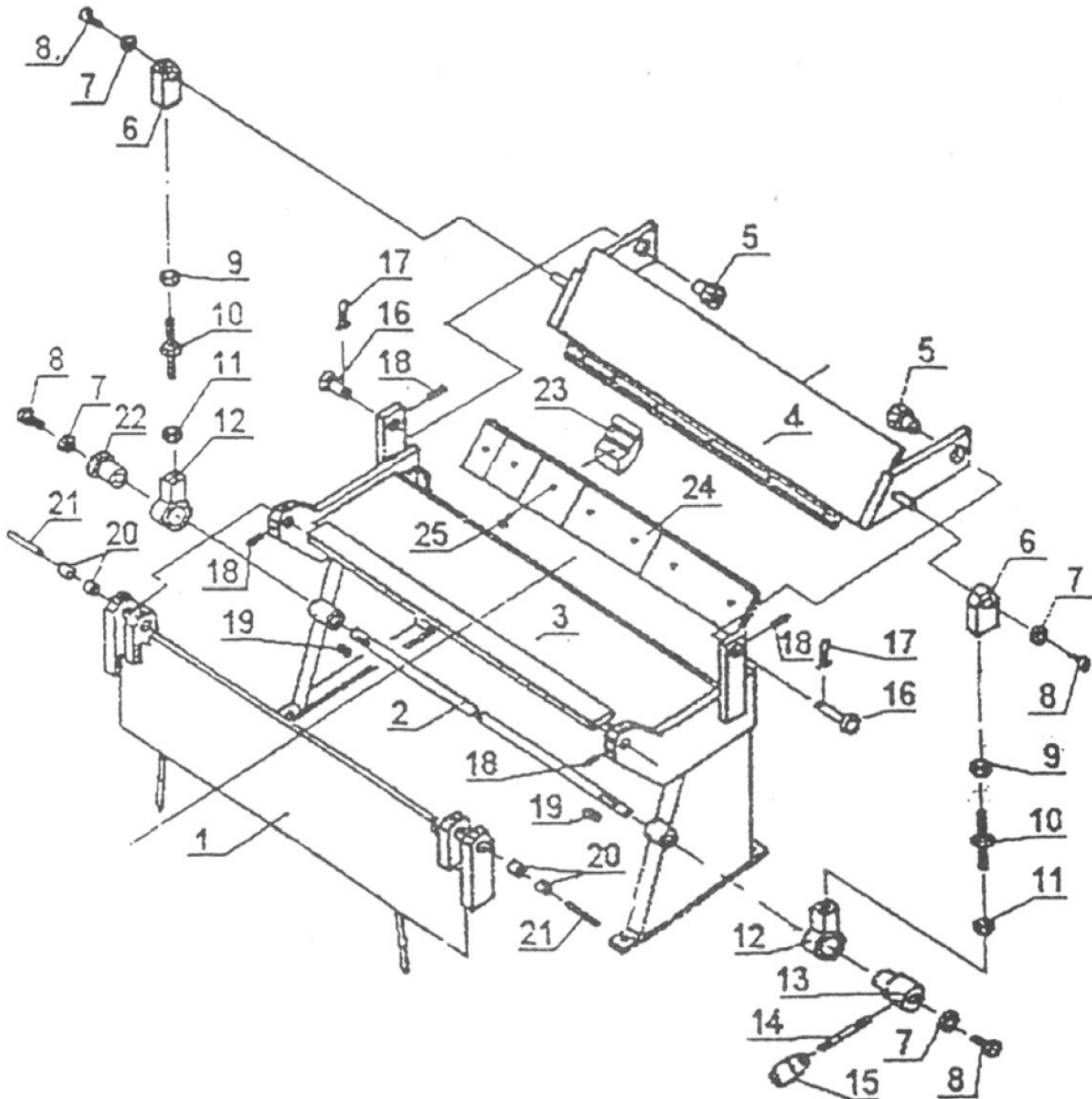
Abb. 8: Ersatzteilzeichnung
