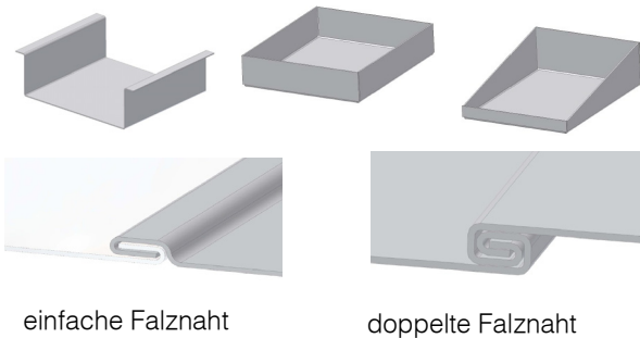
Abb. 6: diverse Biegemöglichkeiten
