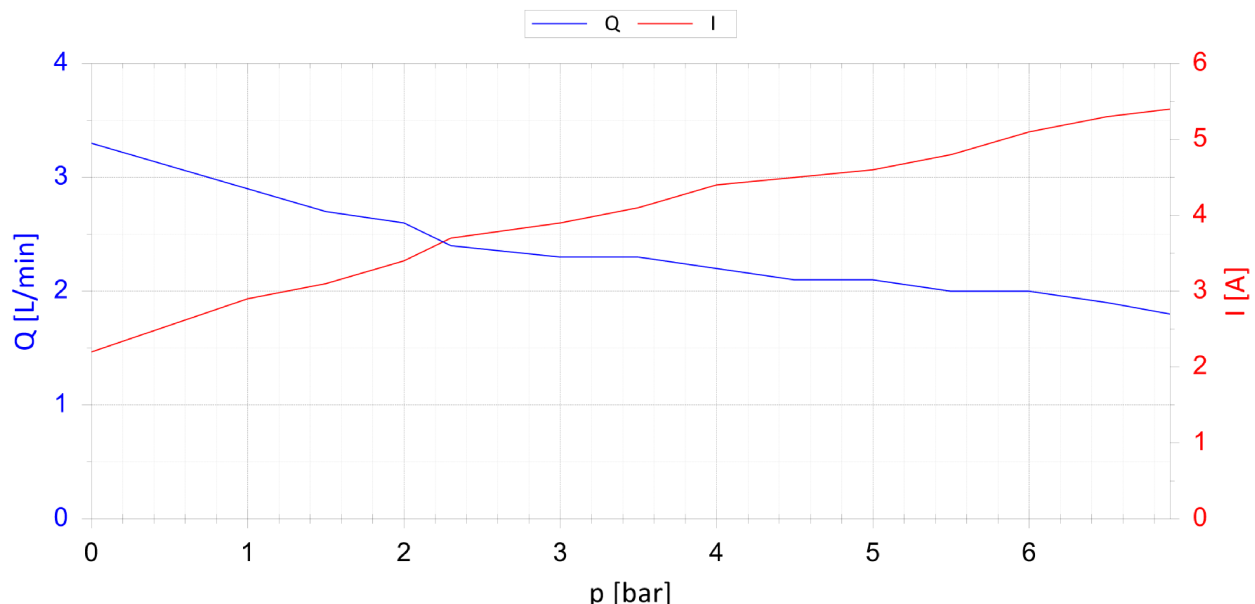
Pumpenkennlinie EM407
